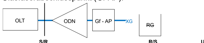
Abbildung 2: XGS-PON auf G.fast Adaption
