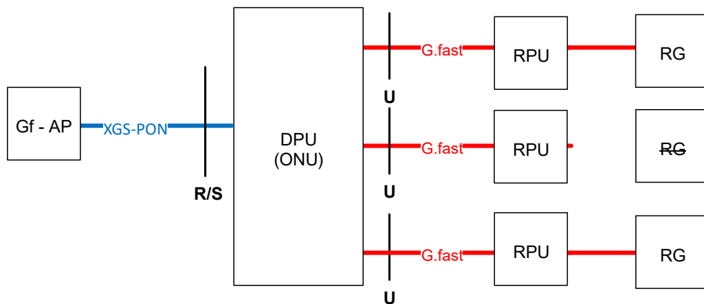
Abbildung 3: Schnittstellen und Netzabschlusspunkt am Kundenstandort
