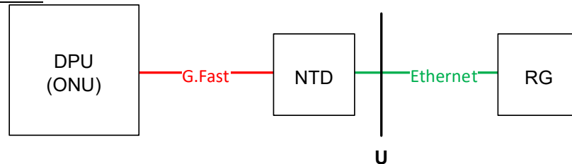
Abbildung 8: U-Schnittstelle NTD
