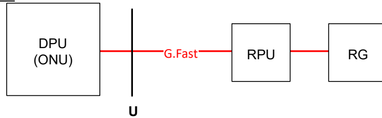
Abbildung 7: U-Schnittstelle RPU
