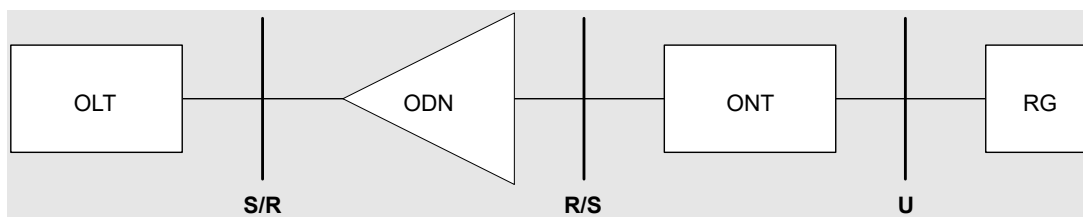
Abbildung 1: Reference points FTTH
